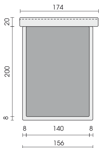
Bed 140 cm Z14
