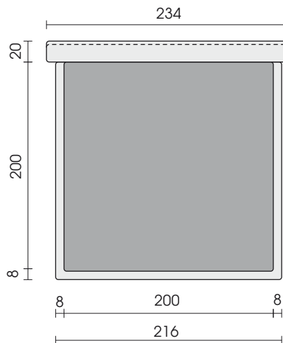
Bed 200 cm Z20
