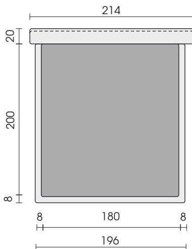
Bed 180 cm B18
